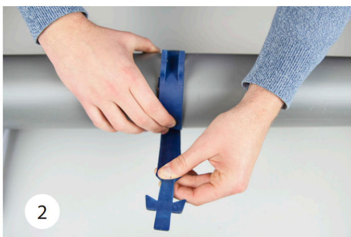
2. Hydra Pipe Strap skal monteres i senter av vegg. Dra litt i enden av Hydra Pipe Strap for å få festet stroppen godt rundt røret
